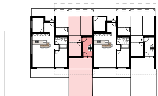
PLAN REZ DE CHAUSSEE
