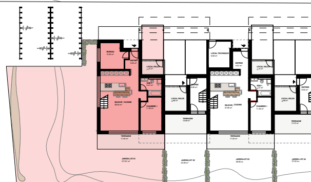
PLAN REZ DE CHAUSSEE
